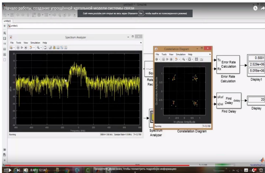
Рисунок 6 - Запуск прогона базовой модели системы тропосферной связи
