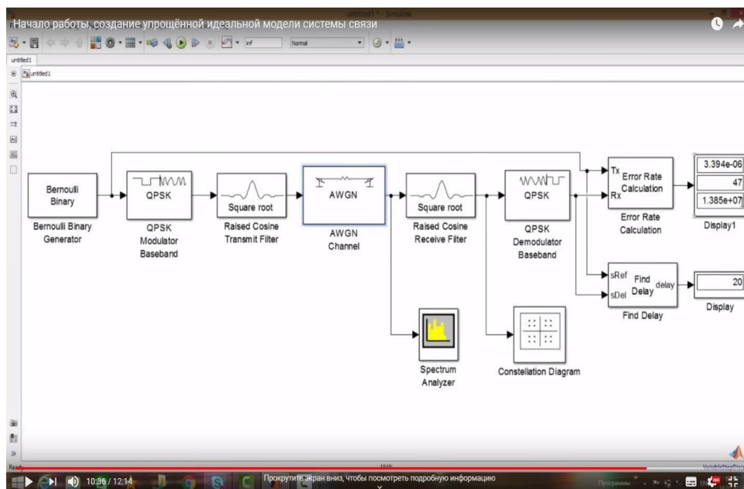
Рисунок 8 - Накопление статистических данных для оценки работы базовой модели CTC
