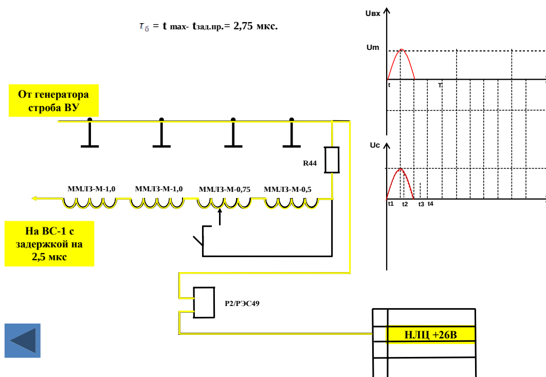
Рисунок 3 - Упрощенная принципиальная схема линии задержки видеоусилителя с ММЛЗ (3,25 мкс)
